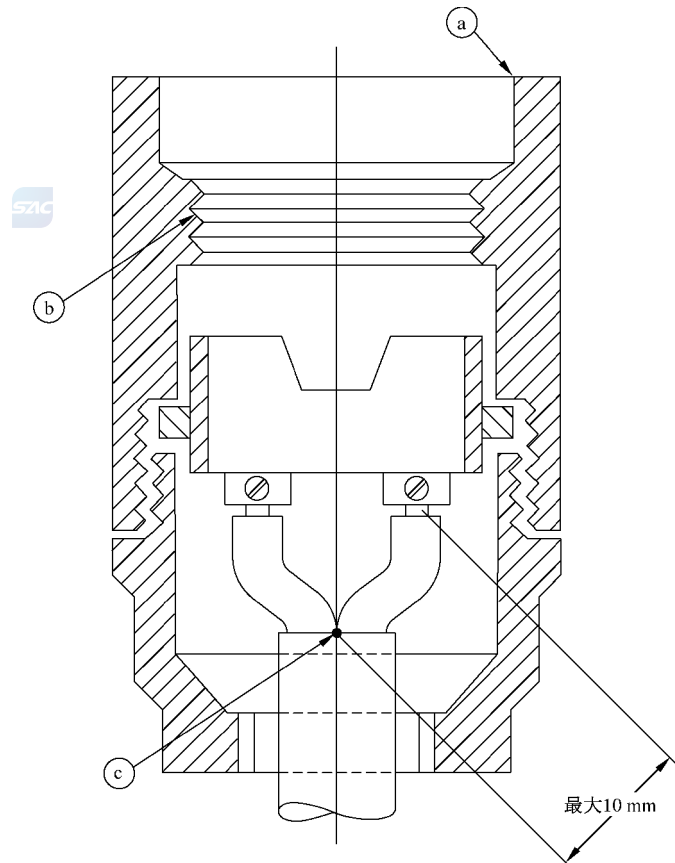
图 K.1 一个典型灯座上热电偶的布置
