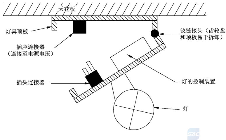
图 31 插头/插座连接的电气-机械接触系统
