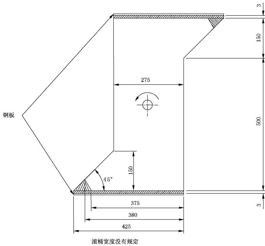
图 25 滚桶
